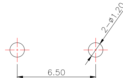
PCB.焊接图
