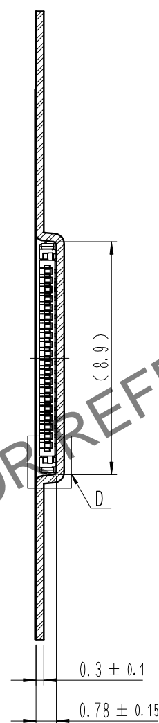
D (10:1)
