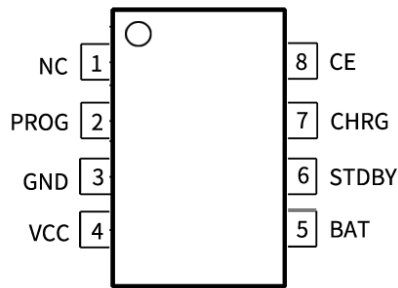
ESOP8
