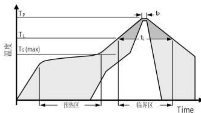
图9 JEDEC 标准的焊接过程图， T_p \leq 260^\circ\text{C} ， t_p < 30\text{sec} ，无铅焊接。 T_L < 220^\circ\text{C} ， t_1 < 150\text{sec} ，焊接时温度上升和下降的速度应 < 5^\circ\text{C}/\text{sec} 。
