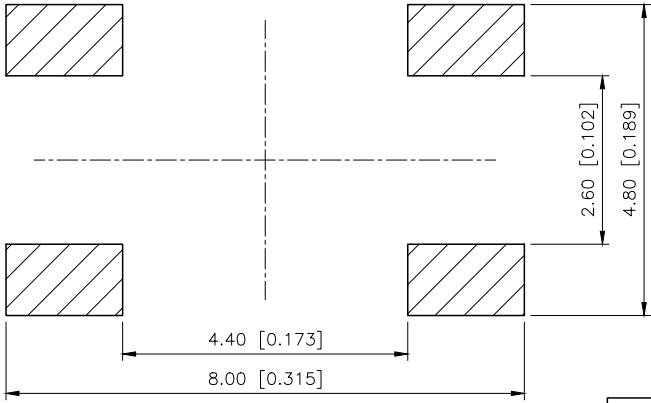
P.C.B LAYOUT
