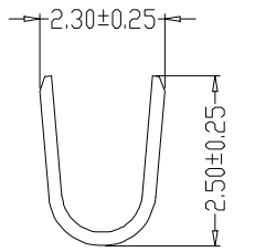
SEC:A-A
