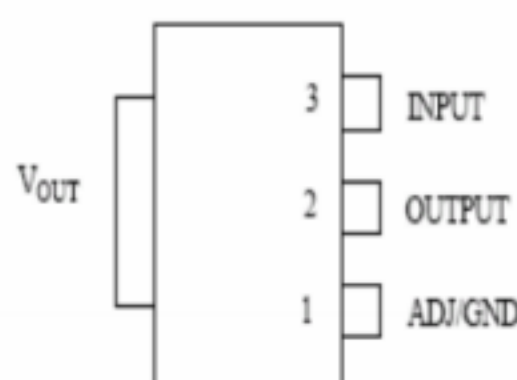
SOT-223
