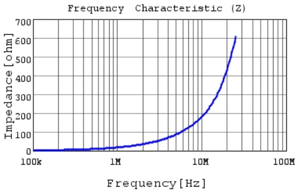
LQM2MPZ3R3NG0 |Z|
