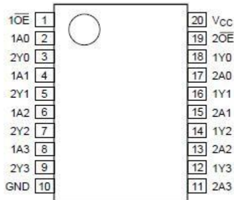
图 2、引脚排列图
