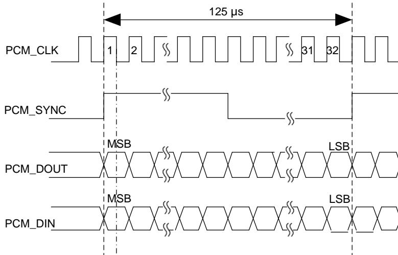
图 25: 长帧模式时序图
