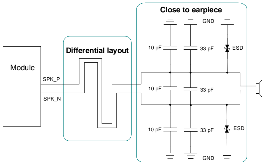
图 28: 听筒输出参考电路
