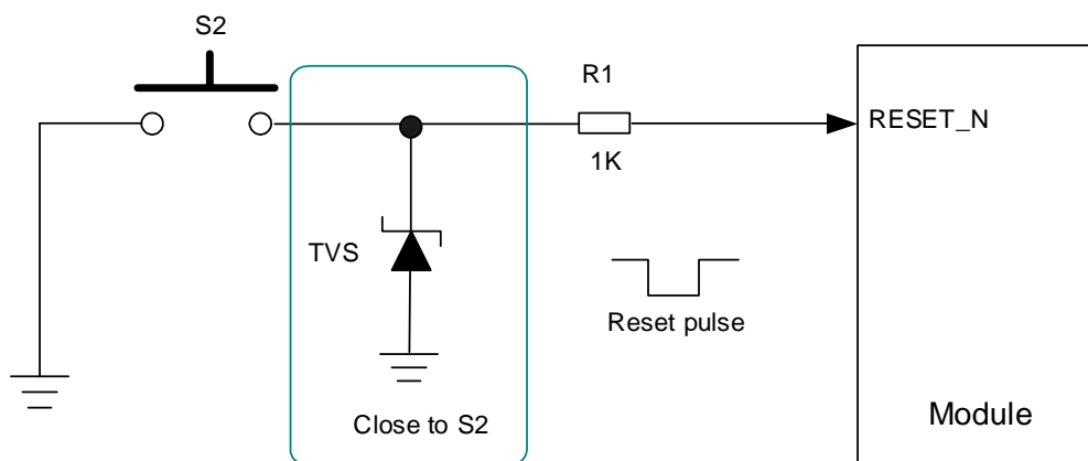
图 15: RESET_N 按键复位参考电路
