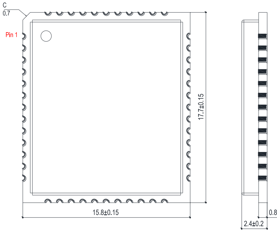
图 42: 模块俯视图及侧视图尺寸图 (单位: mm)
