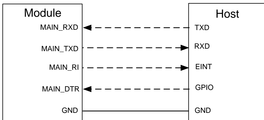
图 3：UART 休眠应用
