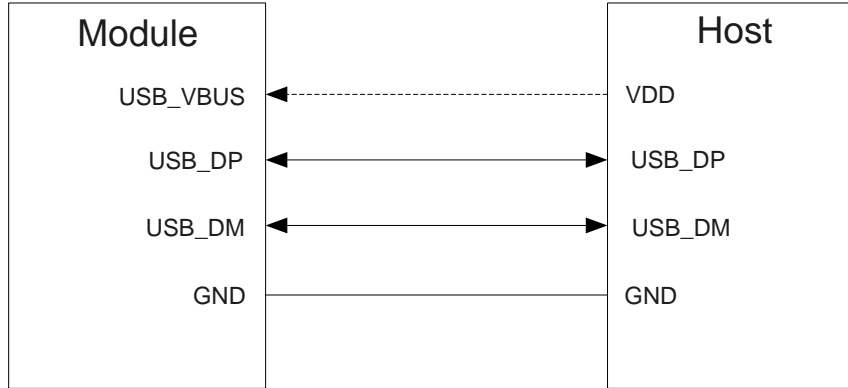
图 4：带 USB 远程唤醒功能的休眠应用
