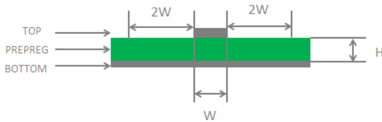
图 35: 两层 PCB 板微带线结构
