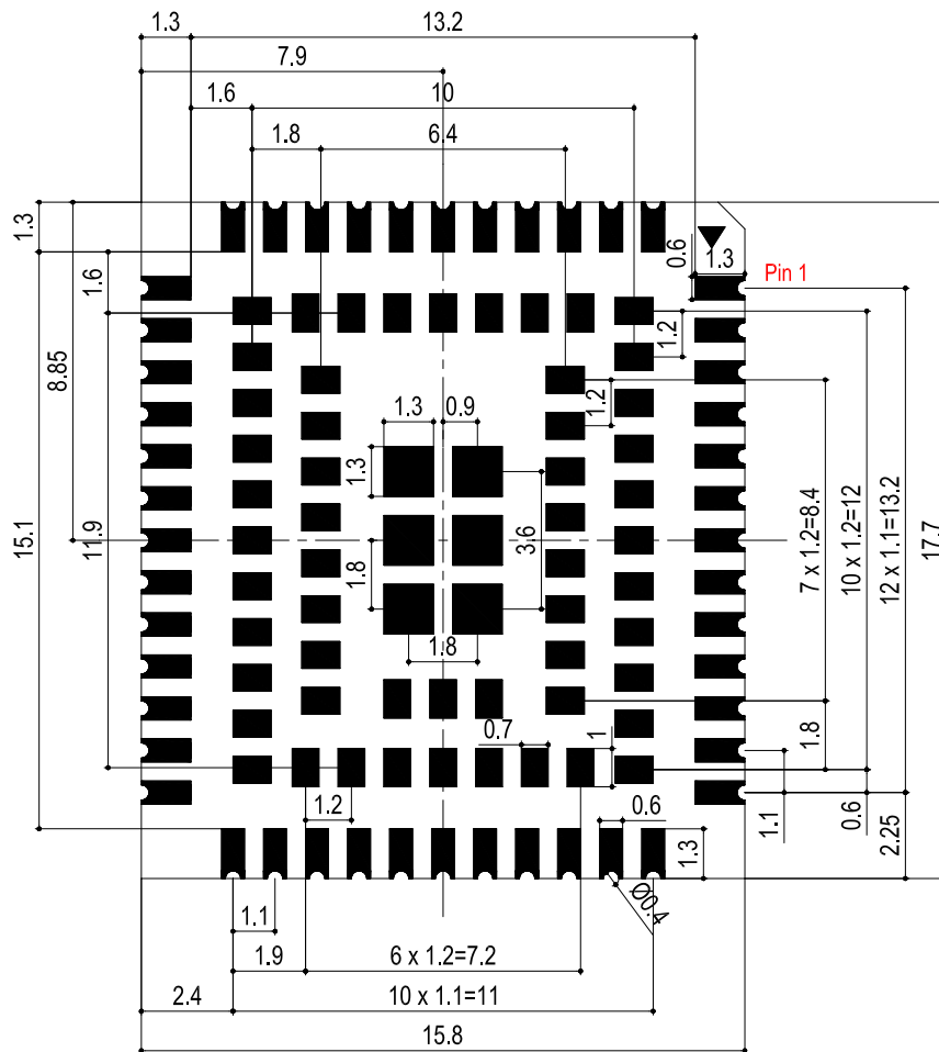
图 43: 模块底视尺寸图
