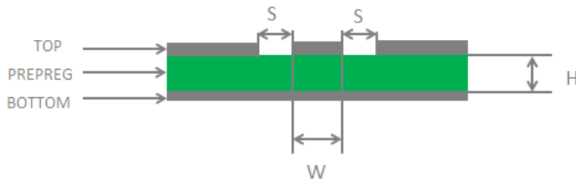
图 36: 两层 PCB 板共面波导结构
