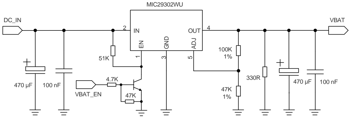
图 7：供电输入参考电路图
