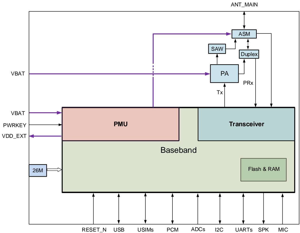
图 1: 功能框图
