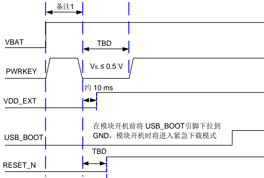
图 19：进入强制下载模式的时序
