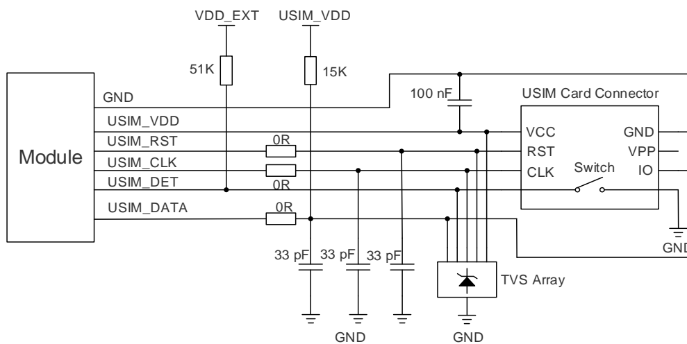
图 20: 8-pin USIM 接口参考电路图
