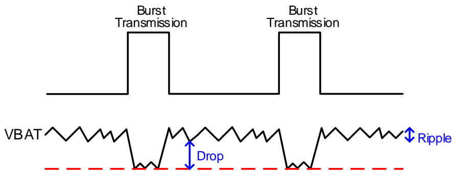
图 8：突发传输电源要求
