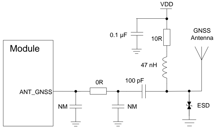
图 33: GNSS 有源天线参考电路
