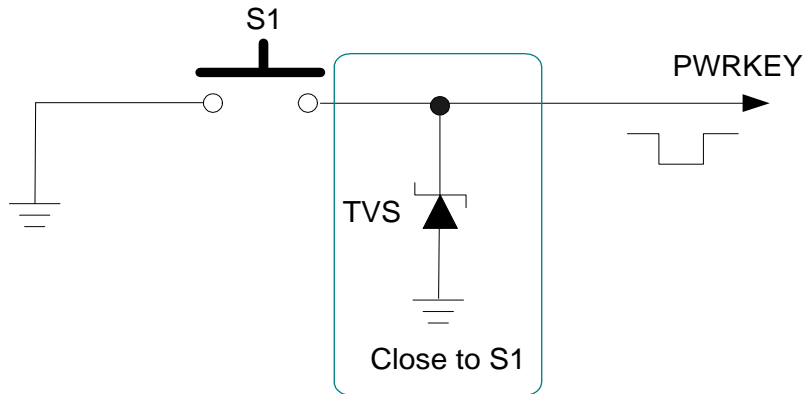
图 11：按键开机参考设计框图
