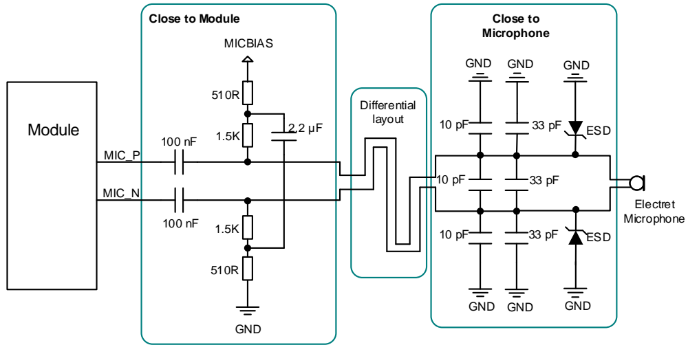
图 27: 麦克风接口参考电路
