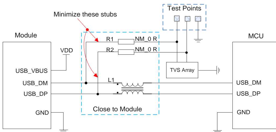
图 17: USB 接口参考设计
