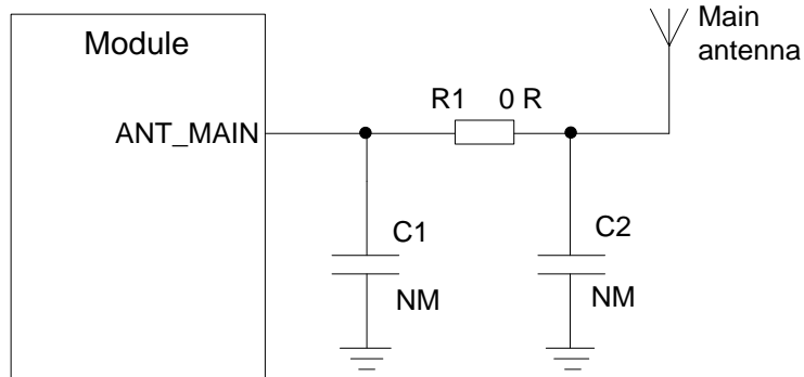
图 32: 射频参考电路图
