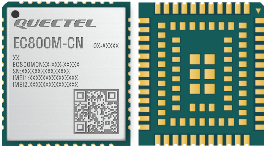
图 45: 模块俯视图和底视图
