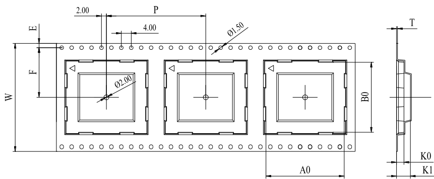
图 47：载带尺寸图
