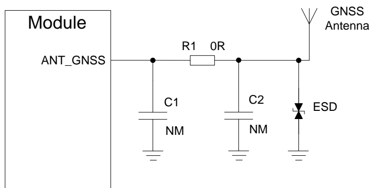
图 34: GNSS 无源天线参考电路
