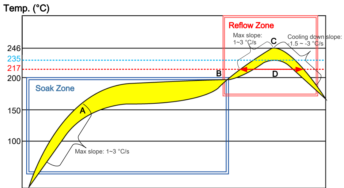
图 46：推荐的回流焊温度曲线
