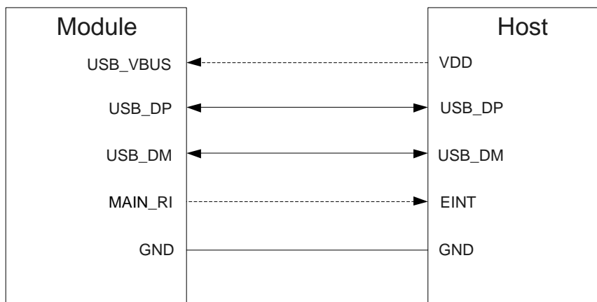
图 5：带 MAIN_RI 功能的休眠应用
