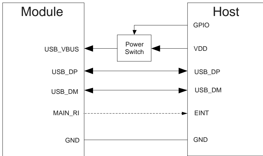
图 6：不支持 USB 挂起功能的休眠应用
