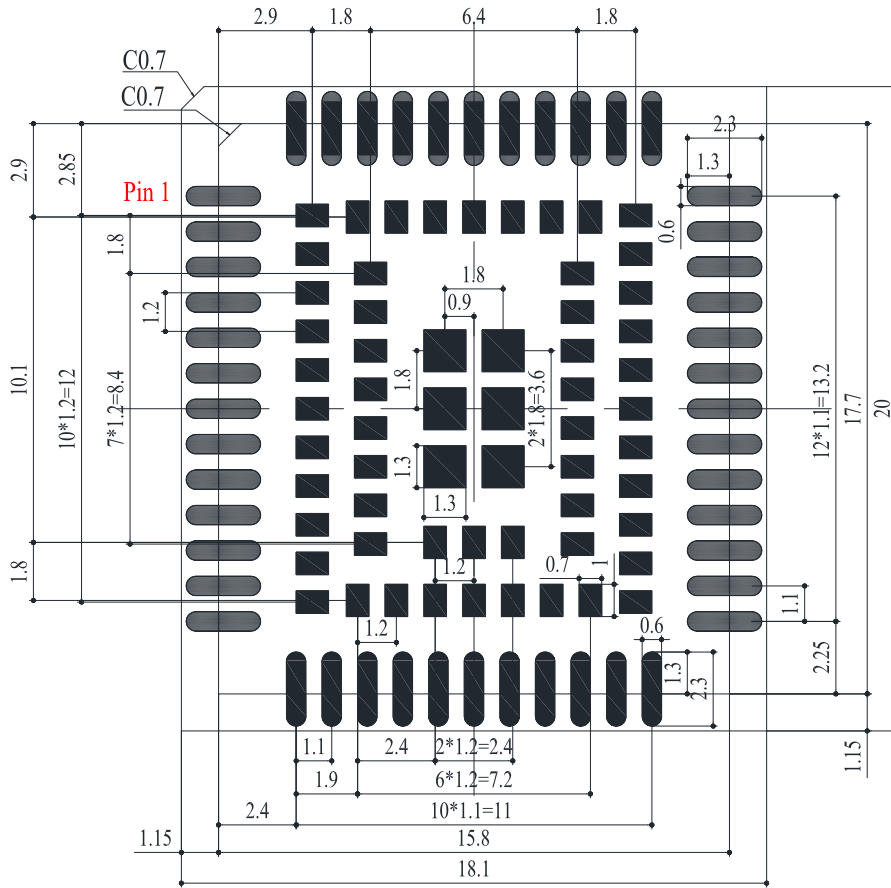
图 44: 推荐封装
