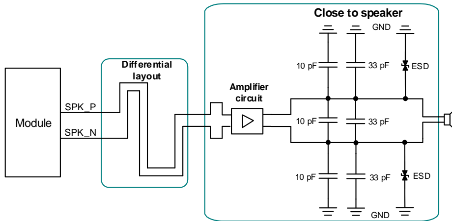
图 29: 扬声器接口参考电路
