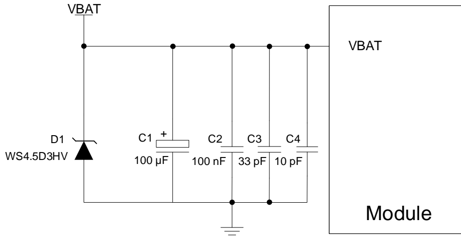
图 9: 模块供电参考电路图
