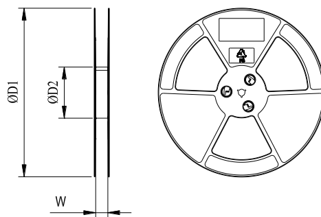
图 48：胶盘尺寸图
