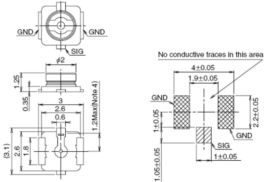
图 39: 天线座尺寸 (单位: mm)
