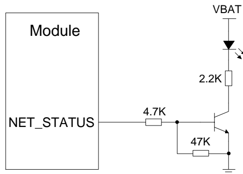
图 30: 网络状态指示参考电路图
