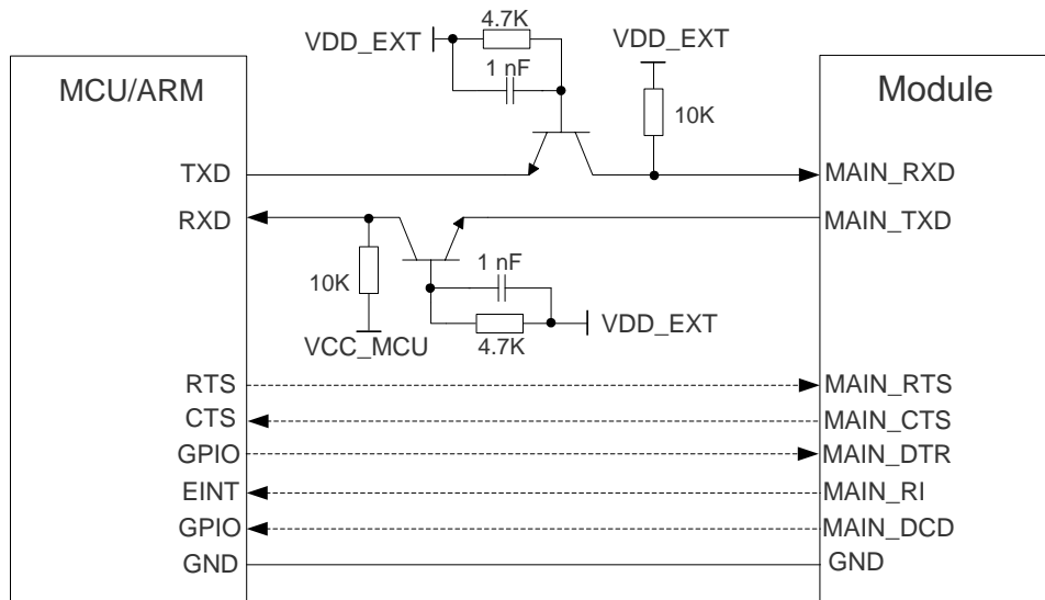
图 23: 电平转换电路参考设计
