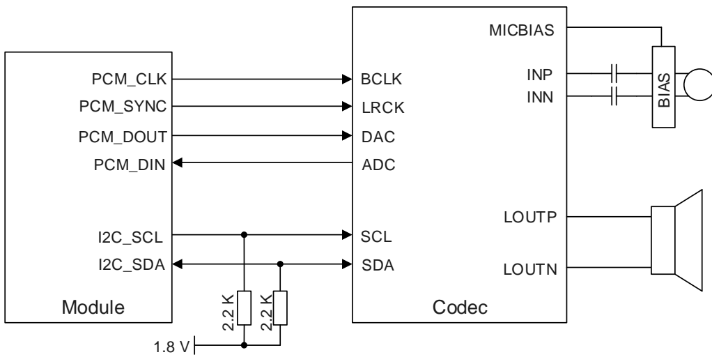
图 26: PCM 和 I2C 接口电路参考设计
