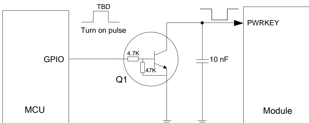
图 10: 开集驱动开机参考设计框图
