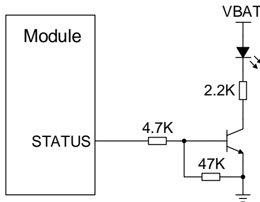
图 31: STATUS 参考电路图
