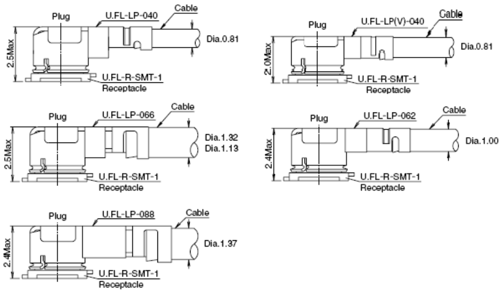
图 41：射频连接器安装图（单位：mm）
