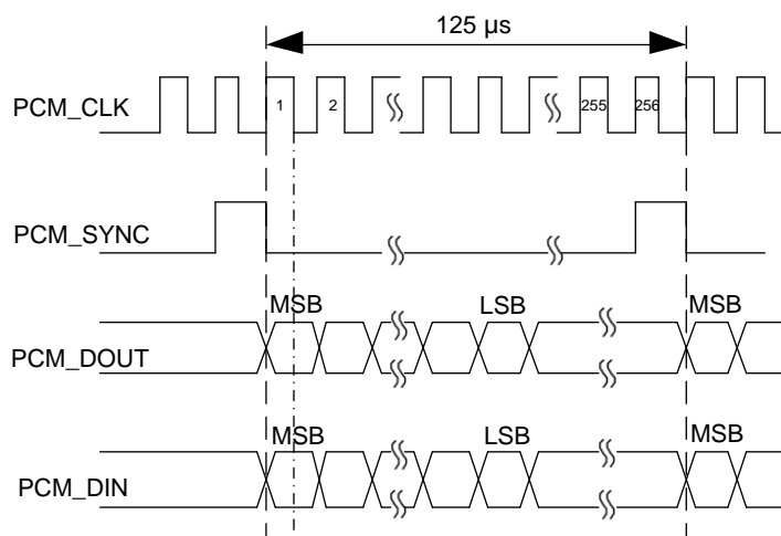
图 24：短帧模式时序图
