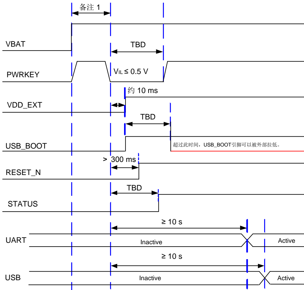
图 12：开机时序图
