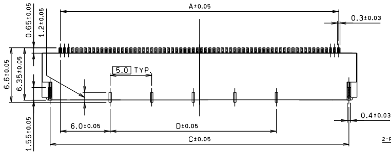
推奨パターン寸法 RECOMMENDED PATTERN LAYOUT
