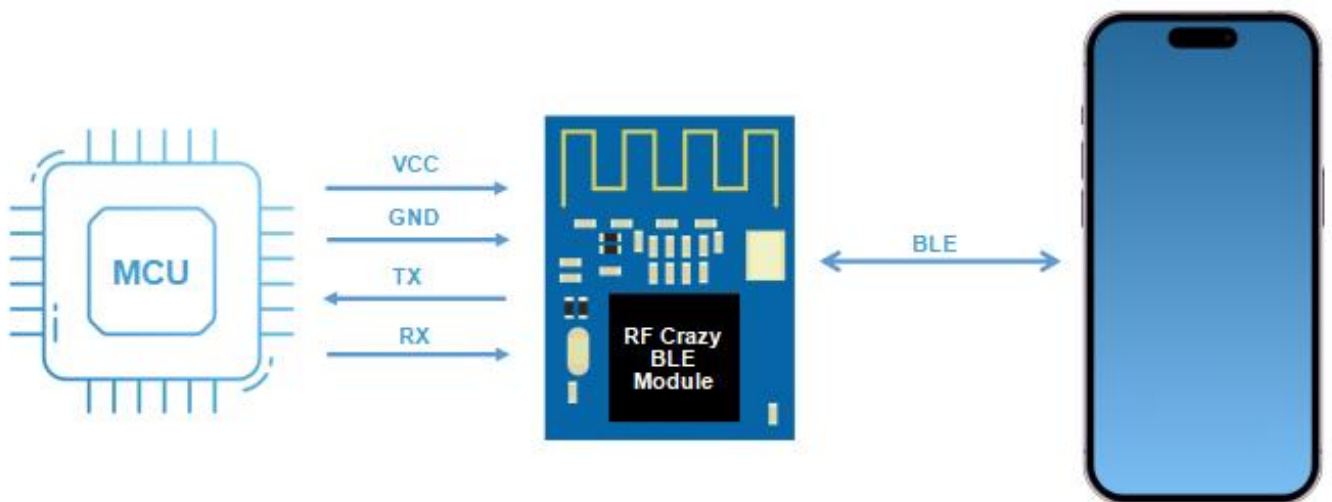
图 2 模块桥接模式示意图
