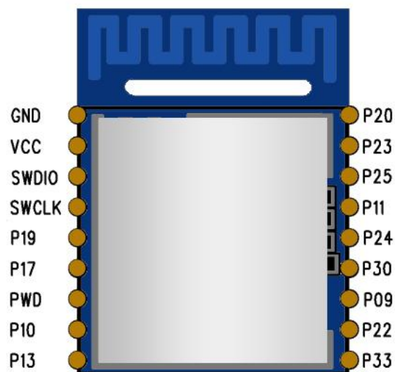
图 4 模块引脚定义图
