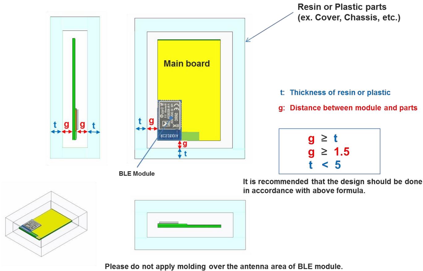
图 8 在树脂或塑胶零部件周围的放置位置
