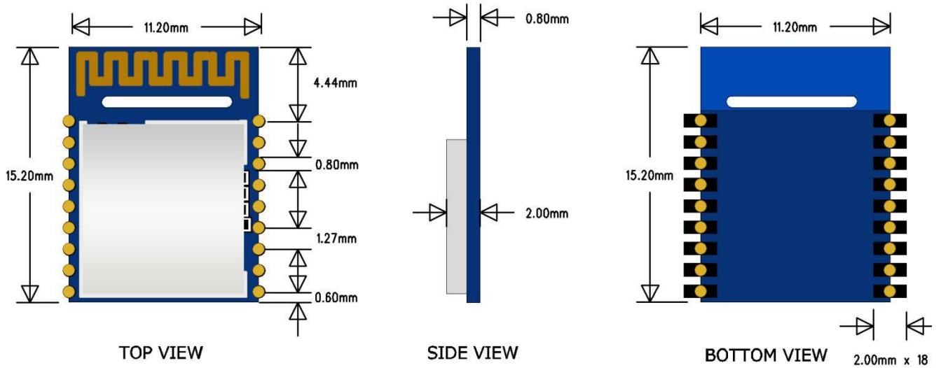
图 3 模块尺寸图
