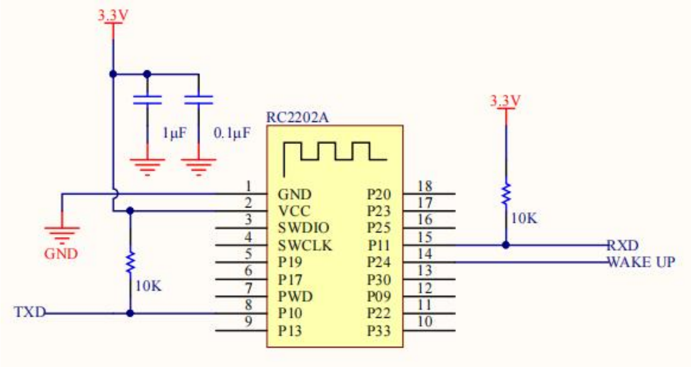
图 5 模块外围推荐电路
