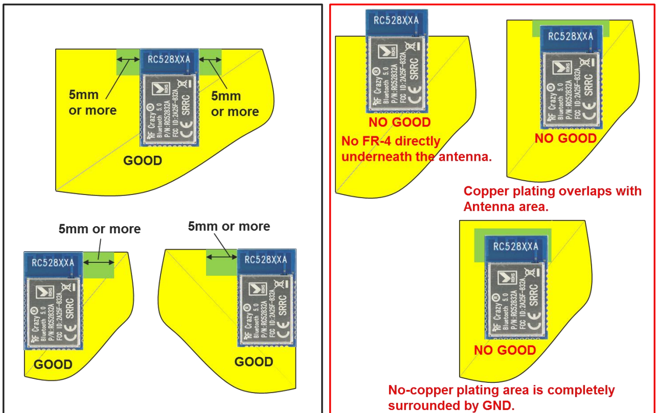
图 7 其他的天线布局建议
