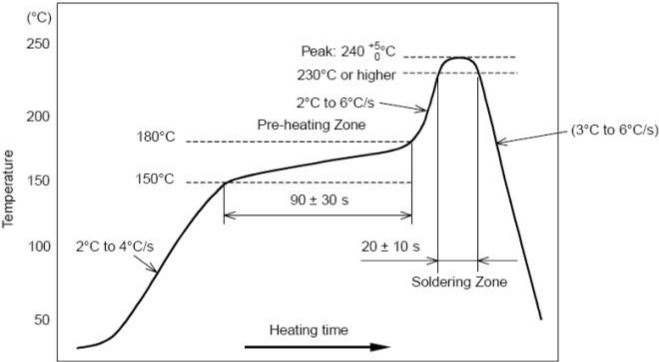
图 9 部件的焊接耐热性温度曲线（焊接点）
