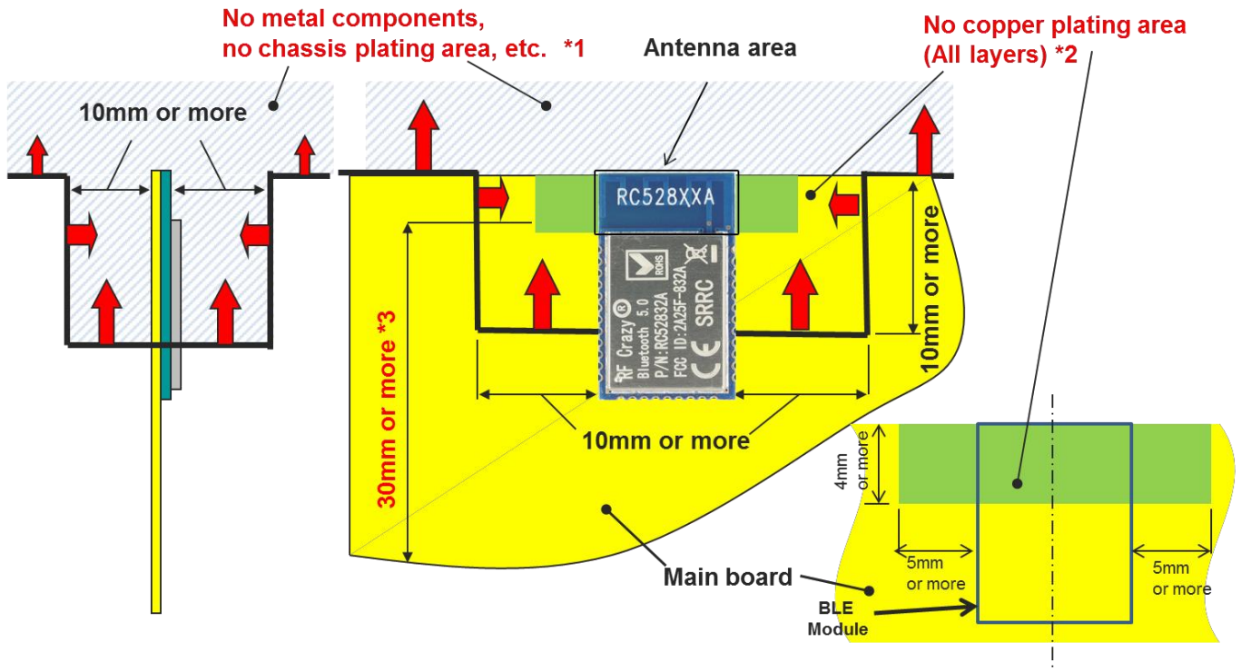
图 6 模块天线布局建议
