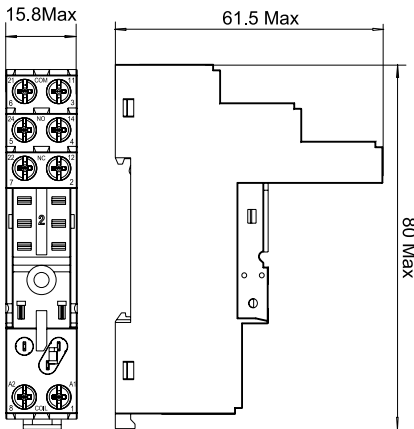
Dimensions : Millimetres
