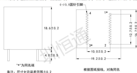
主视图
