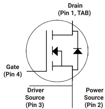
TO-247-4
