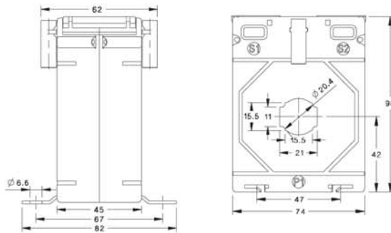
XMER 74-30
