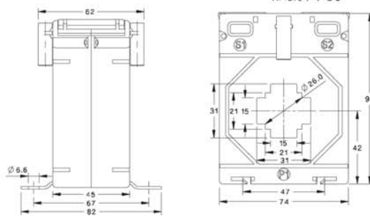
XMER 74-40
