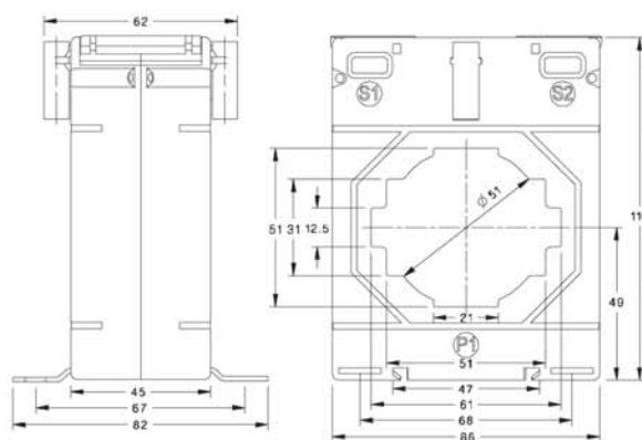
XMER 86-60
