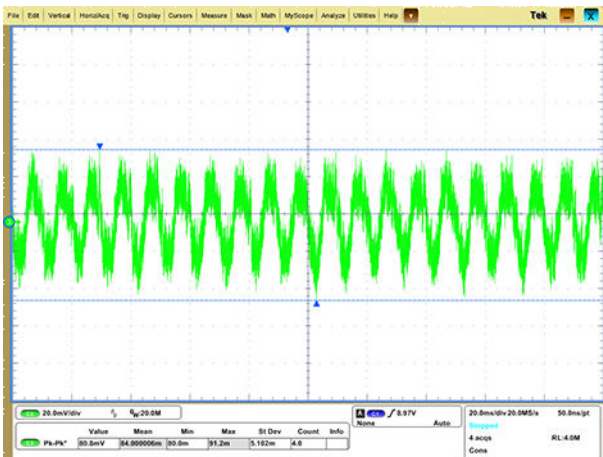
输出电压纹波 ( V_{in}=220V AC)
