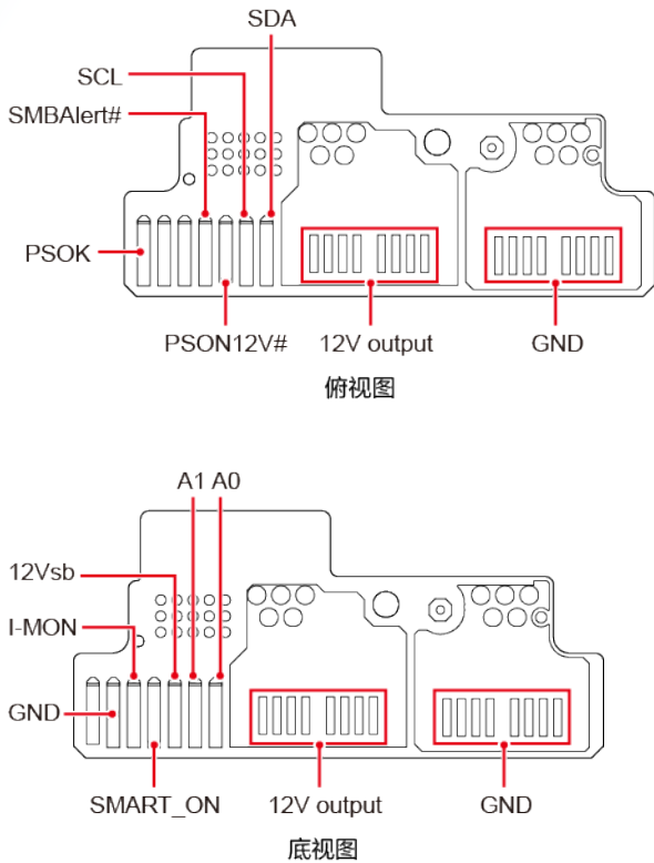
图 4-2 端子介绍
