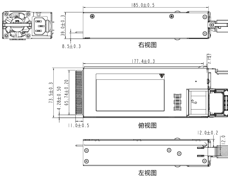
图 4-1 结构尺寸
