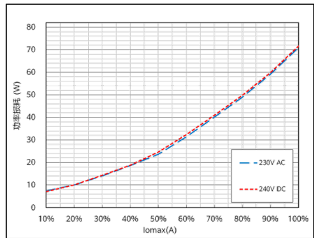
功率损耗曲线（不带风扇）
