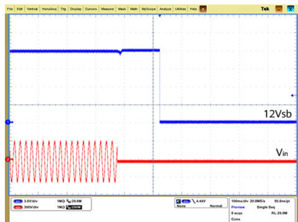
关机 ( V_{in}=220\text{V DC} , V_{out}=12\text{Vsb} )
