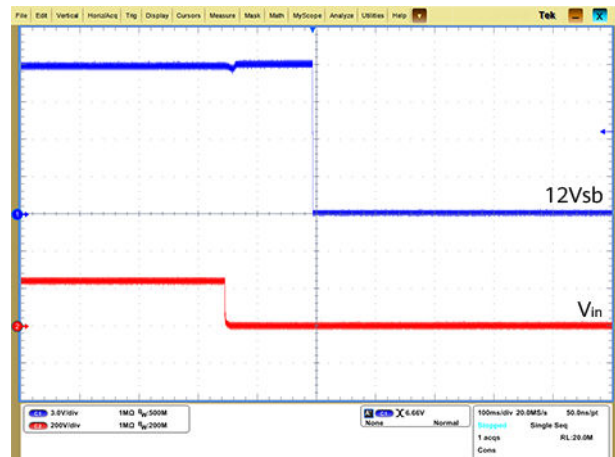
关机 ( V_{in}=240V DC, V_{out}=12Vsb )
