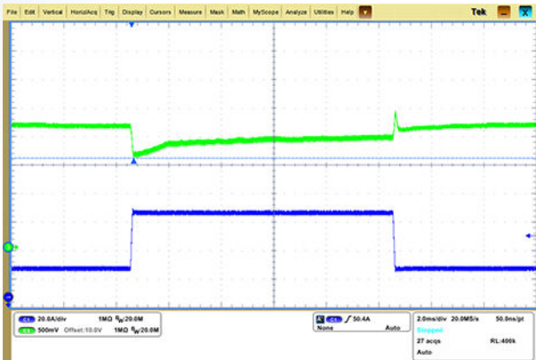
输出电压动态响应
