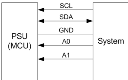
图 11-1 I2C 接口
