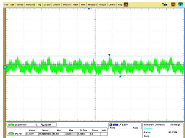
输出电压纹波 ( V_{in}=240V DC)
