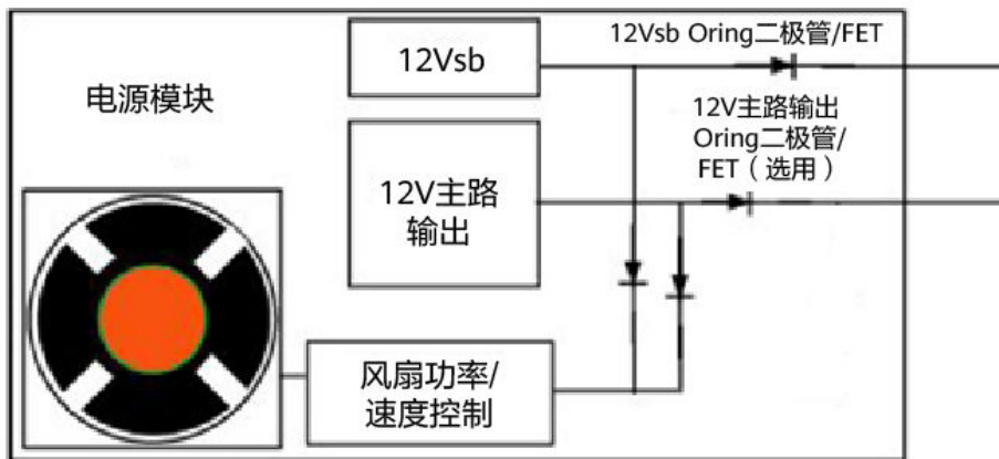
图 12-1 风扇供电电路图
