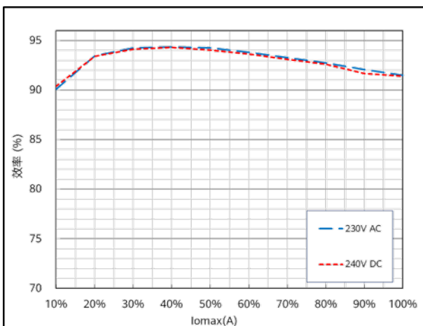
效率曲线（带风扇）
