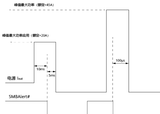
图 3-1 峰值功率时序图
