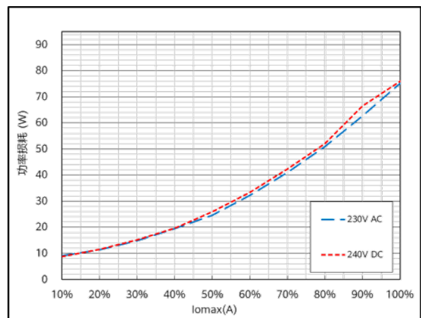
功率损耗曲线（带风扇）
