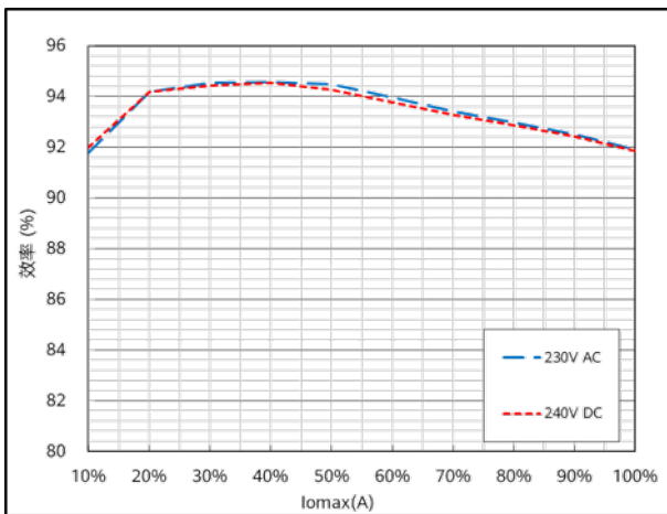
效率曲线（不带风扇）
