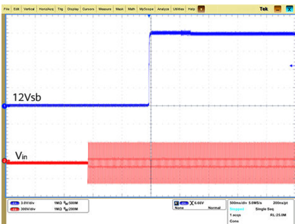
开机 ( V_{in}=220\text{V DC} , V_{out}=12\text{Vsb} )
