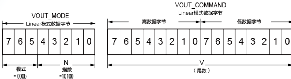
图 11-4 VOUT 数据格式
