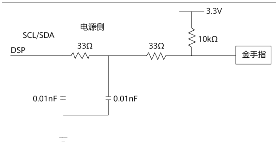
图 11-2 SCL 与 SDA 对接示意图
