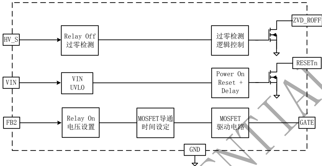
图 3 BP8009 内部框图
