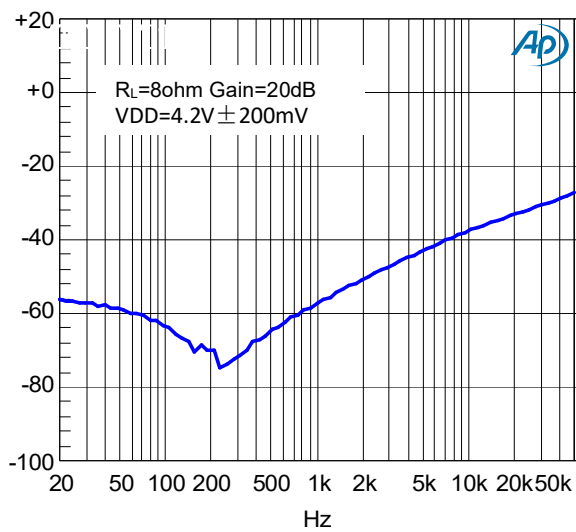
PSRR
