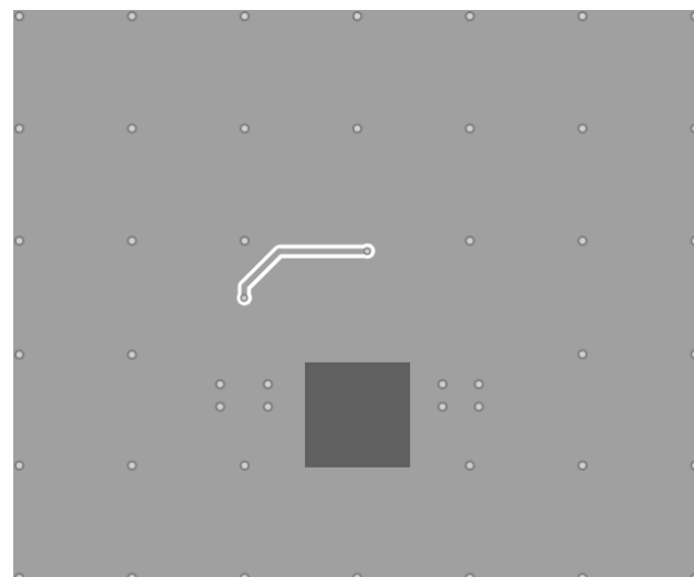
Bottom Layer
