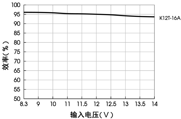
效率Vs输入电压 ( V_{out}=5V, I_o=16A )
