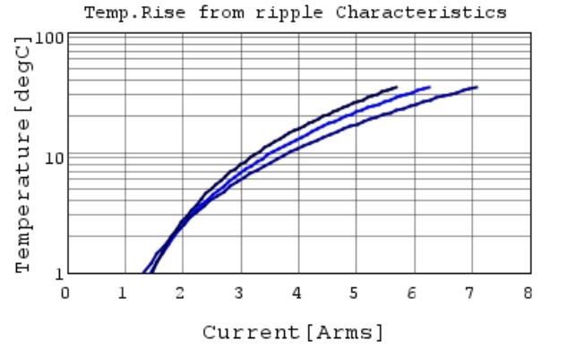
GCM32EC7YA106KA03 Temp.rise — 80kHz
